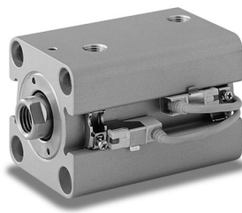
CBY14シリーズ薄形シリンダ
