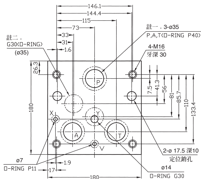
■ ELFB(C)G-06 安裝尺寸
