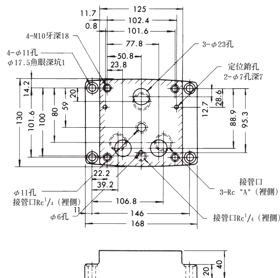
底板 EFBGM-03Y, 03Z-10
