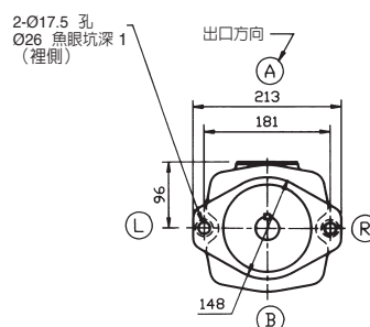
腳架安裝型
