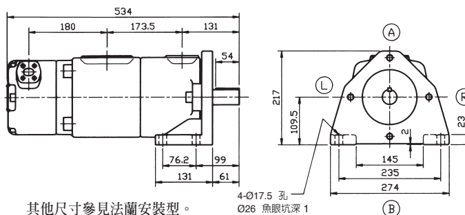
腳架安裝型
