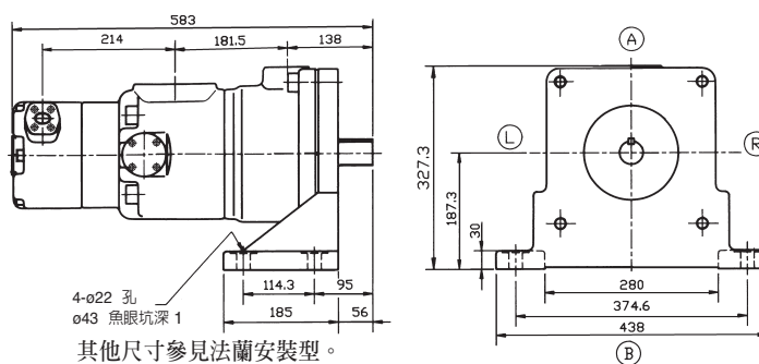
腳架安裝型
