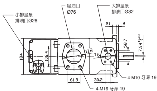
法蘭安裝型
