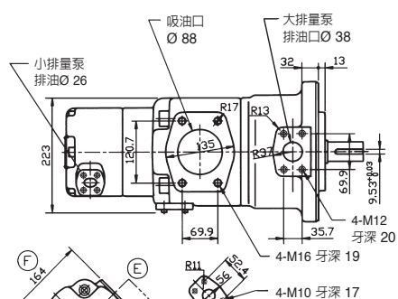
法蘭安裝型
