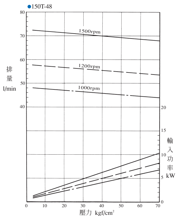
壓力—排量，輸入功率特性 作動油黏度20cSt
