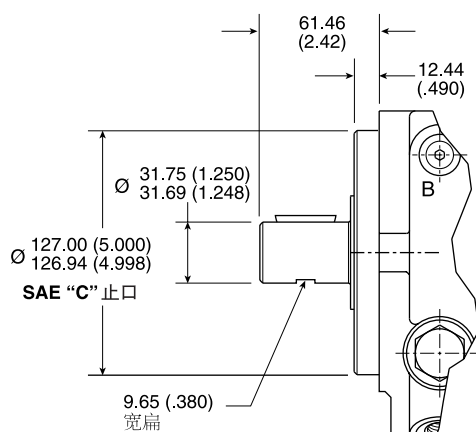
SAE "C" 止口 1-1/4" (31.75) 直径 5/16" (7.9) 平键轴
