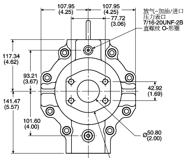
后进油口 (进口选项 "省略") 见油口尺寸表
