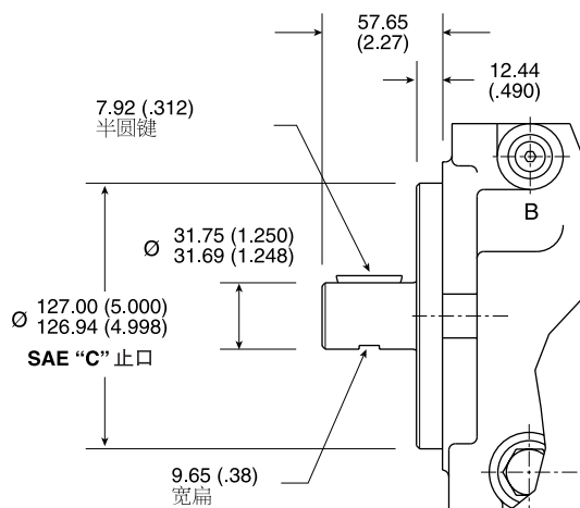
SAE "C" 止口 1-1/4" (31.75) 直径 5/16" (7.9) 平键轴
